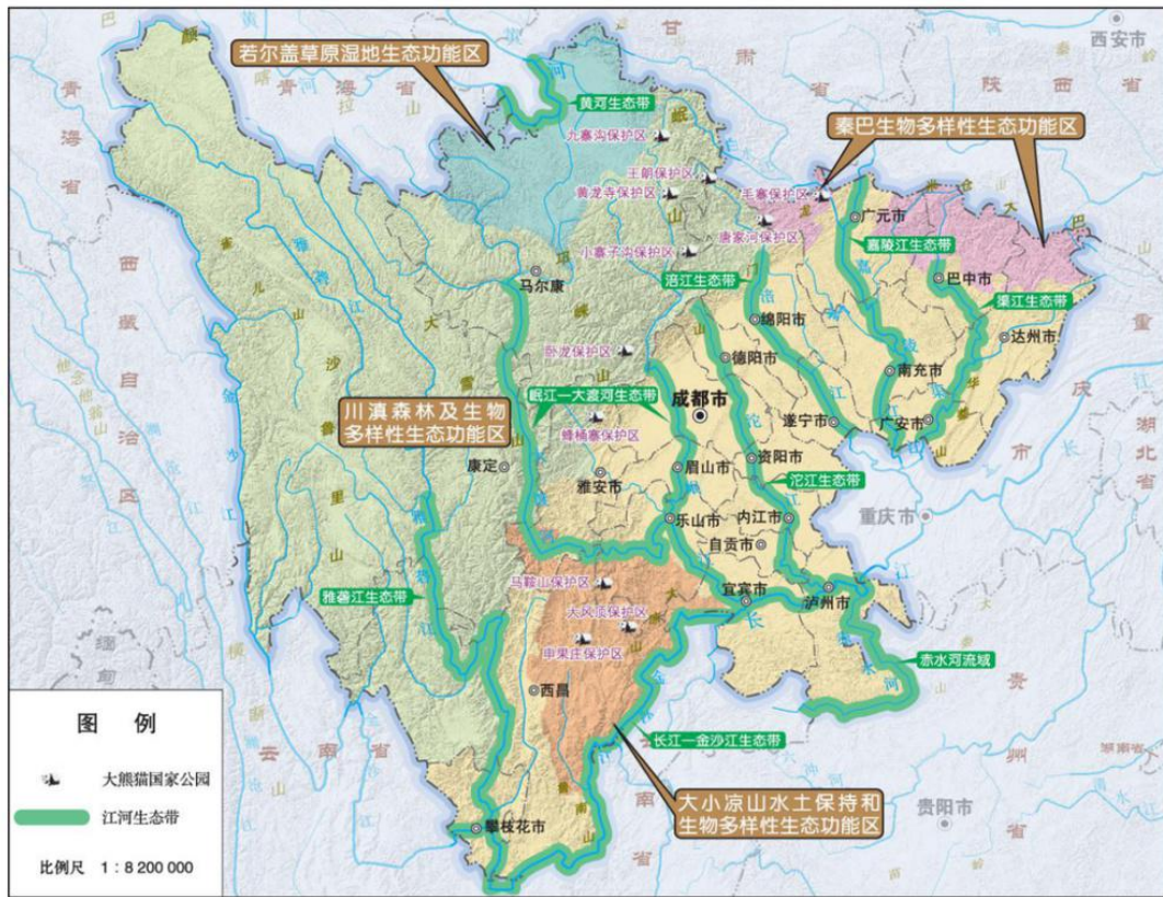
图 5 生态安全格局示意图
